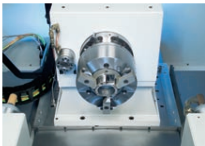
SK 204 凸轮磨床的加工区 带修整器的头架
