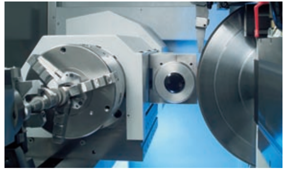
动力驱动的金刚石修整轮正在修整陶瓷粘结的 CBN 砂轮
